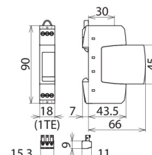
Maßbild DR M 2P 30 FM
