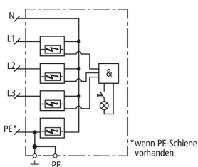
Prinzipschaltbild DV ZP TT 255
