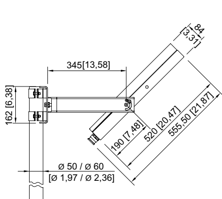
Scheinwerfer mit Mastbefestigung
