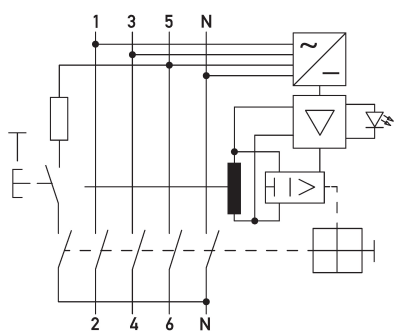
Schaltungsbeispiel Fehlerstromschutzschalter DFS 4 040-4/0,30-PV R HD
