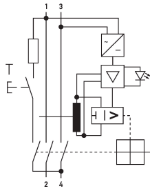
Schaltungsbeispiel Fehlerstromschutzschalter DFS 2 025-2/0,30-PV
