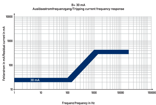
Diagramme Fehlerstromschutzschalter DFS 4 040-4/0,03-B+ MI
