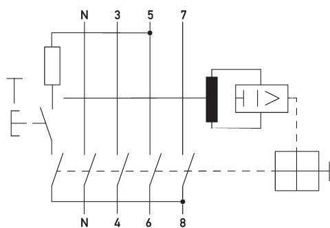
Schaltungsbeispiel Fehlerstromschutzschalter DFS 4 040-4/0,10-A
