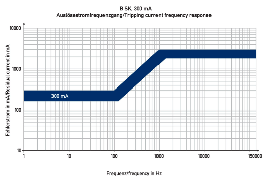
Diagramme Fehlerstromschutzschalter DFS 2 025-2/0,30-B SK
