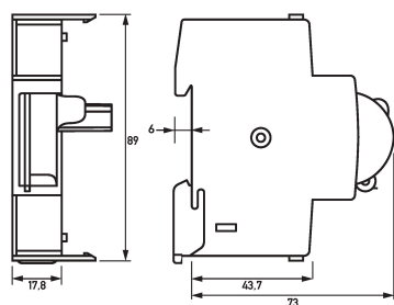
Maßzeichnung Gruppenansicht
