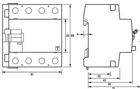
Maßzeichnung Gruppenansicht
