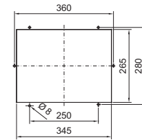
Montaj kesiti
