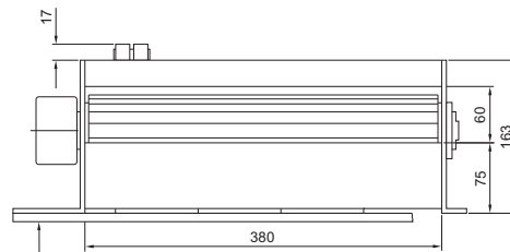
Ön ızgara
