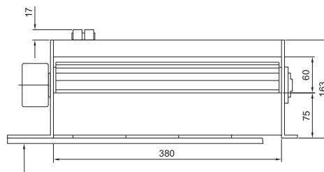
Etupuolen ritilä
