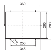
Montageudskæring
