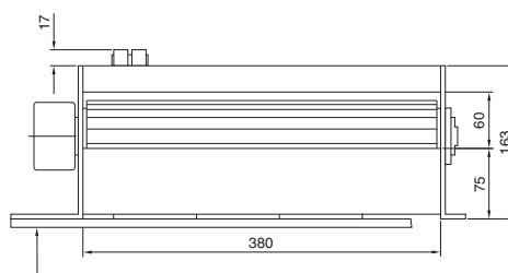
Frontgitter
