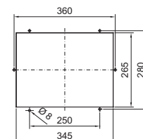
Wykroj montażowy
