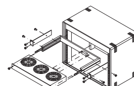
Moduł wentylatorowy wsuwany Vario Montaż na płaszczyźnie 482,6 mm (19")
