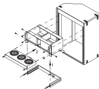
Moduł wentylatorowy wsuwany Vario Montaż we wspornikach podspółów 84 TE
