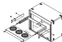
Schuiflade-ventilator Vario Montage in 482,6 mm (19")-systemen
