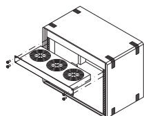
Schuiflade-ventilator Montage in 482,6 mm (19")-systemen
