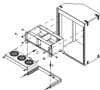
Zásuvné ventilátory Vario Montáž do vany 84 TE
