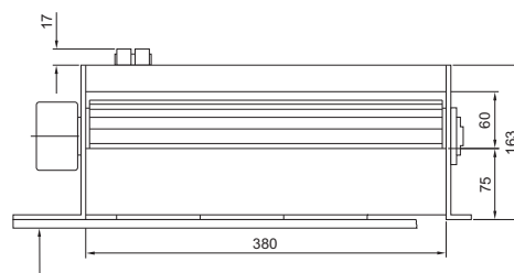
Mřížka na přední straně
