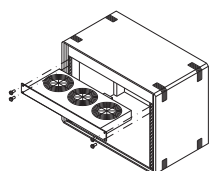
Zásuvné ventilátory Montáž do 482,6 mm (19") roviny
