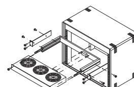
Zásuvné ventilátory Vario Montáž do 482,6 mm (19") roviny
