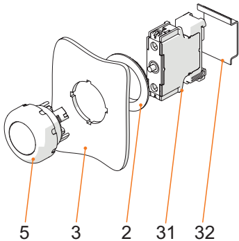
Tragschienenmontage
