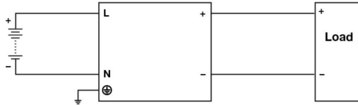
Abb. 4 Anschlussschema für den Betrieb mit Gleichstrom-Eingang
