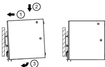
Abb. 3.1 Montage
