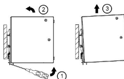
Abb. 3.2 Demontage
