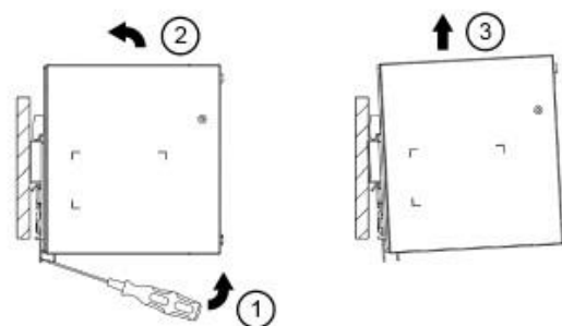
Abb. 3.2 Demontage
