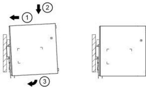
Abb. 3.1 Montage
