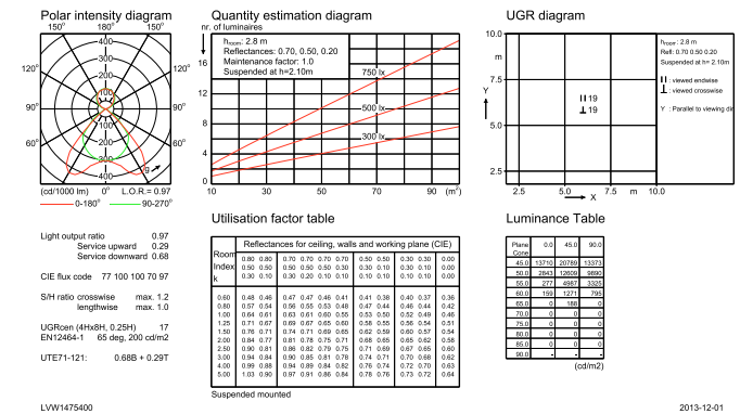
TPS642 1xTL5-54W HFP D8-VH
