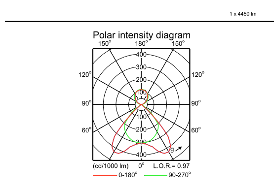
TPS642 1xTL5-54W HFP D8-VH
