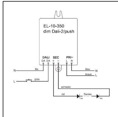
Anschluss dim Push
