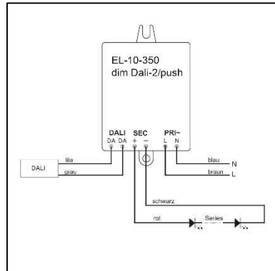
Anschluss dim Dali2
