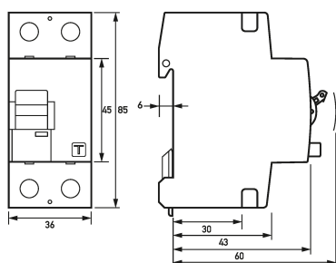
Maßzeichnung Fehlerstromschutzschalter DFS 2 025-2/0,03-HP
