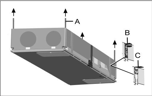
Variantes de fixation [A], [B] ou [C]
