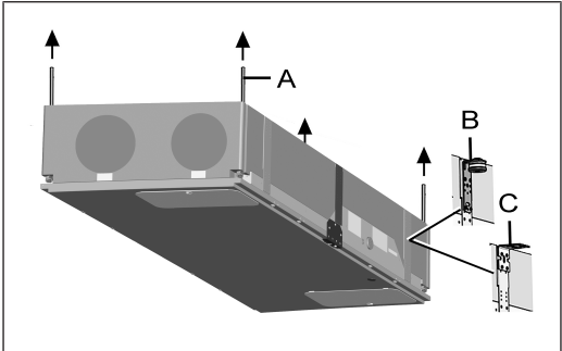
Befestigungsvarianten [A], [B] oder [C]
