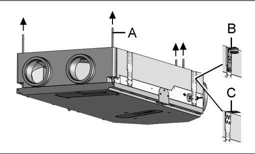
Befestigungsvarianten [A], [B] oder [C]
