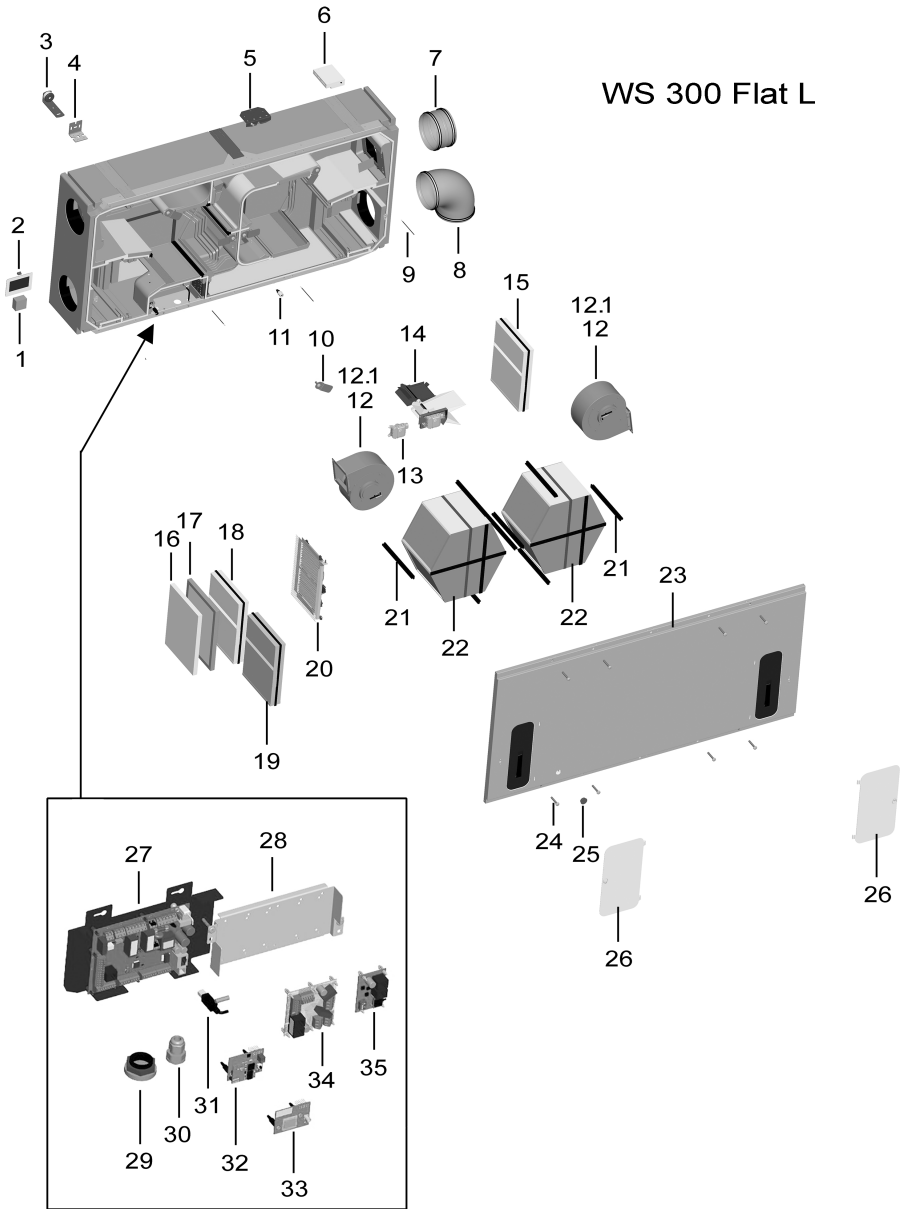
Abbildung = WS 300 Flat L Ohne Abbildung = spiegelbildliche Variante WS 300 Flat R
