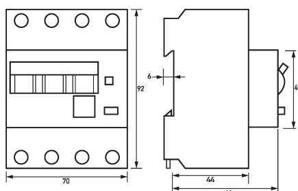
Maßzeichnung FI-/LS-Kombinationen DRCBO 4 B32/0,03/3N-A
