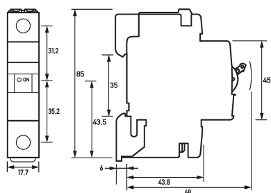
Maßzeichnung Leitungsschutzschalter DLS 6hsl B16-1
