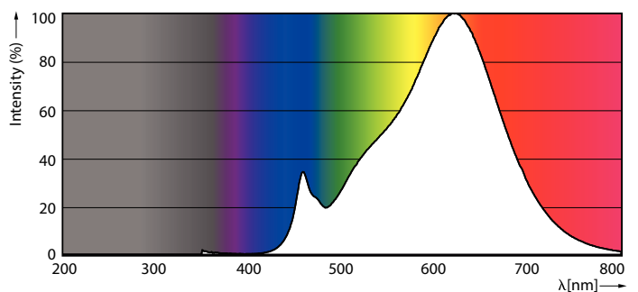
LEDbulb CLA 4,5W B35 E14 927 922 CL
