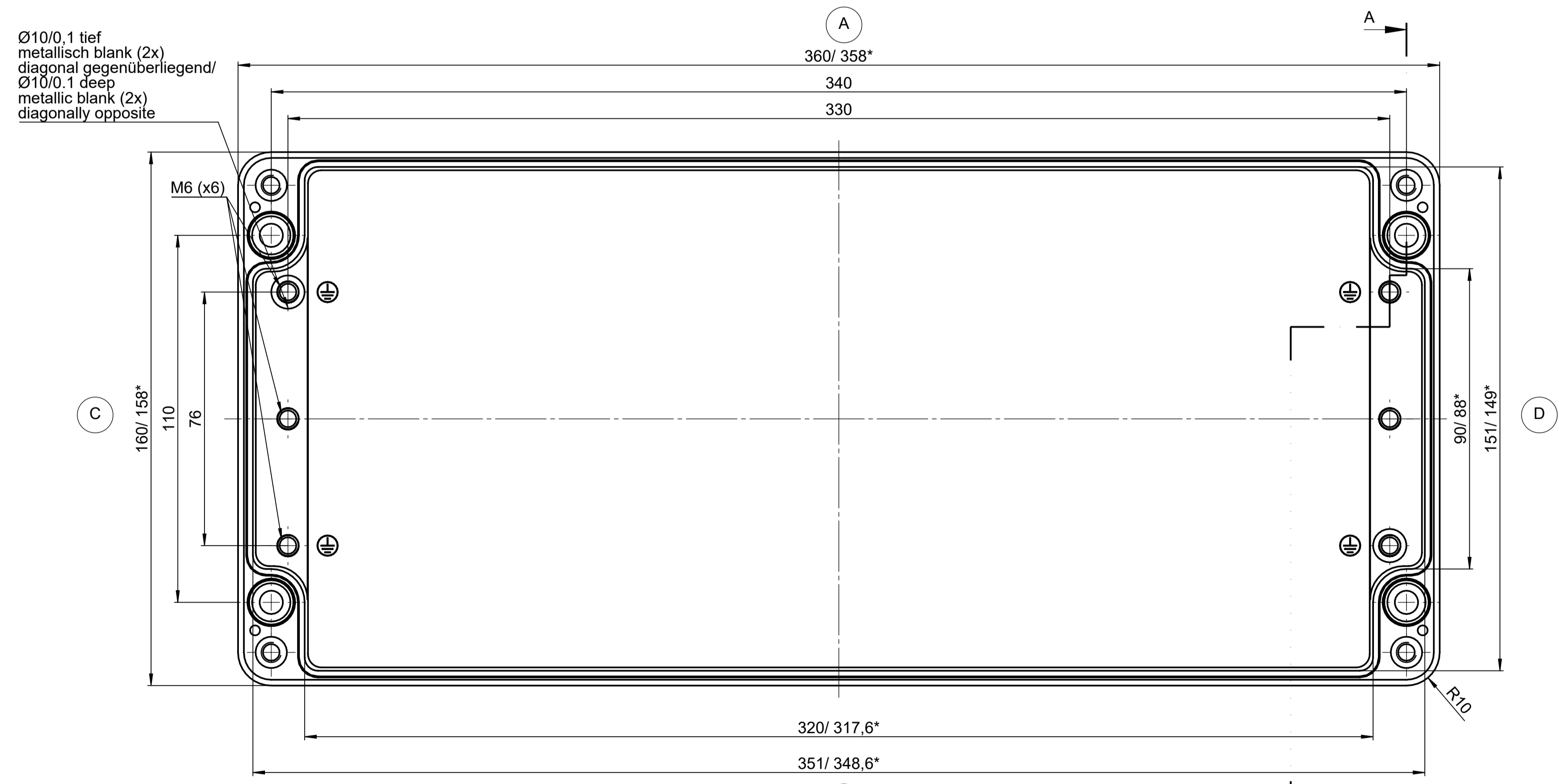
Unterteil / Base
