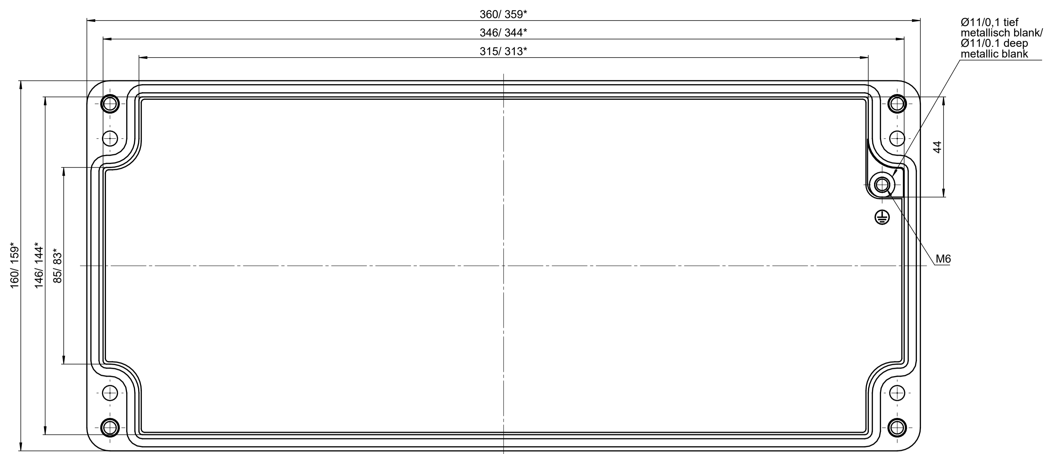
Deckel / Lid
