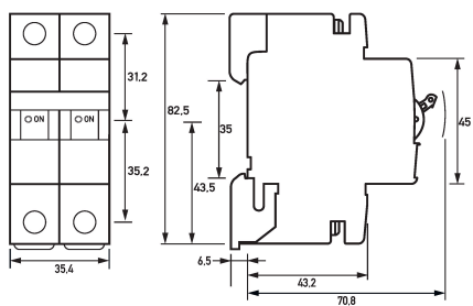
Maßzeichnung Gruppenansicht
