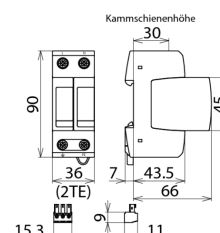
Maßbild DG M TT 2P CI 275 FM
