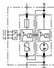
Prinzipschaltbild DG M TT 2P CI 275 FM
