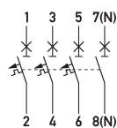
Schaltungsbeispiel Leitungsschutzschalter DLS 6h B25-3+N
