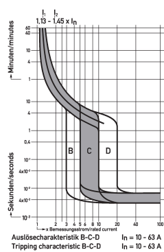
Diagramme Leitungsschutzschalter DLS 6h B25-3+N
