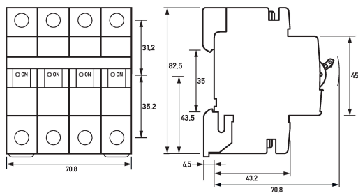
Maßzeichnung Leitungsschutzschalter DLS 6h C13-3+N
