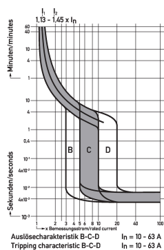
Diagramme Leitungsschutzschalter DLS 6h C13-3+N
