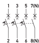
Schaltungsbeispiel Leitungsschutzschalter DLS 6h C13-3+N
