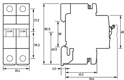
Maßzeichnung Leitungsschutzschalter DLS 6hdc C6-2
