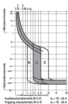
Diagramme Leitungsschutzschalter DLS 6h C25-2
