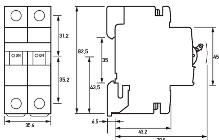
Maßzeichnung Leitungsschutzschalter DLS 6h C25-2
