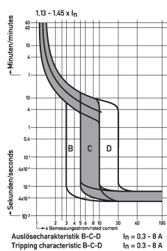
Diagramme Leitungsschutzschalter DLS 6h B6-2
