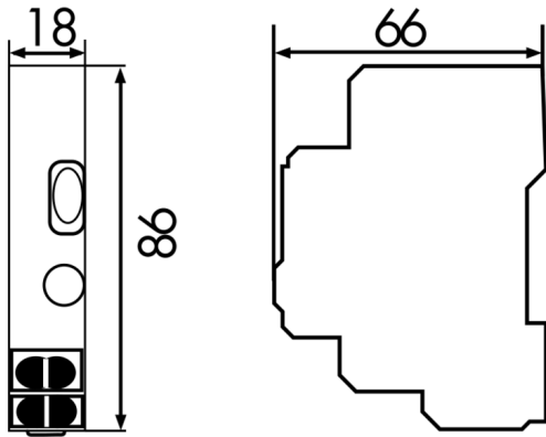
Bemaßung 92655
