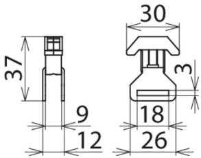
Maßbild AK 35 SN 18X3 GG
