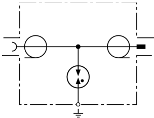
Prinzipialschaltbild DGA G SMA
