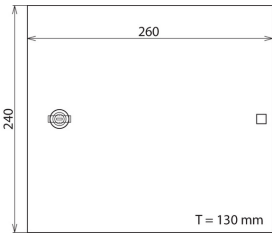
Maßbild DPG LSA 30 P
