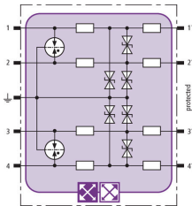
Prinzipschaltbild BXT ML4 BE C 24
