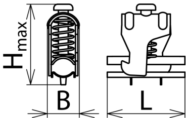
Maßbild SAK
