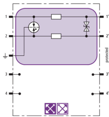
Prinzipialschaltbild BXT ML2 BD 180
