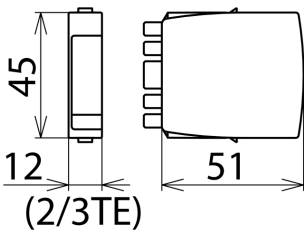
Maßbild BXT ML2 BD 180
