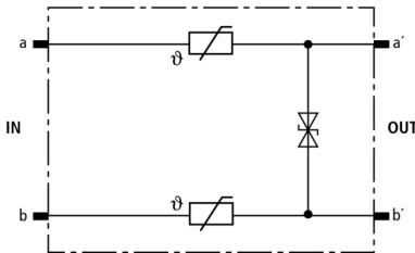
Prinzipschaltbild DRL PD 180
