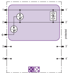
Prinzipschaltbild BXT ML2 BD HF EX 6
