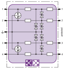
Prinzipialschaltbild BXT ML4 BE C 12
