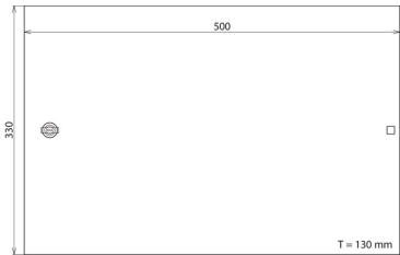
Maßbild DPG LSA 220 P
