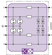
Prinzipschaltbild BXT ML4 BC EX 24
