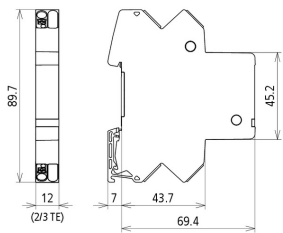
Maßbild BCO CL2 BD HC10A 24
