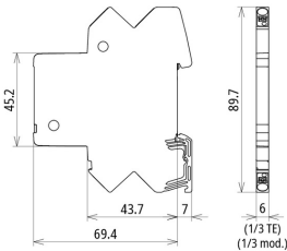
Maßbild BCO CL2 BD EX 24
