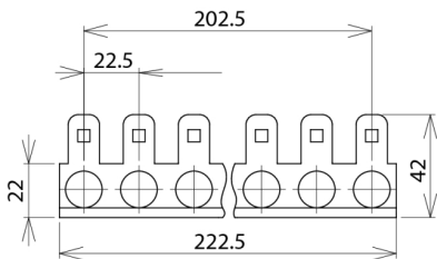
Maßbild MB2 10 LSA
